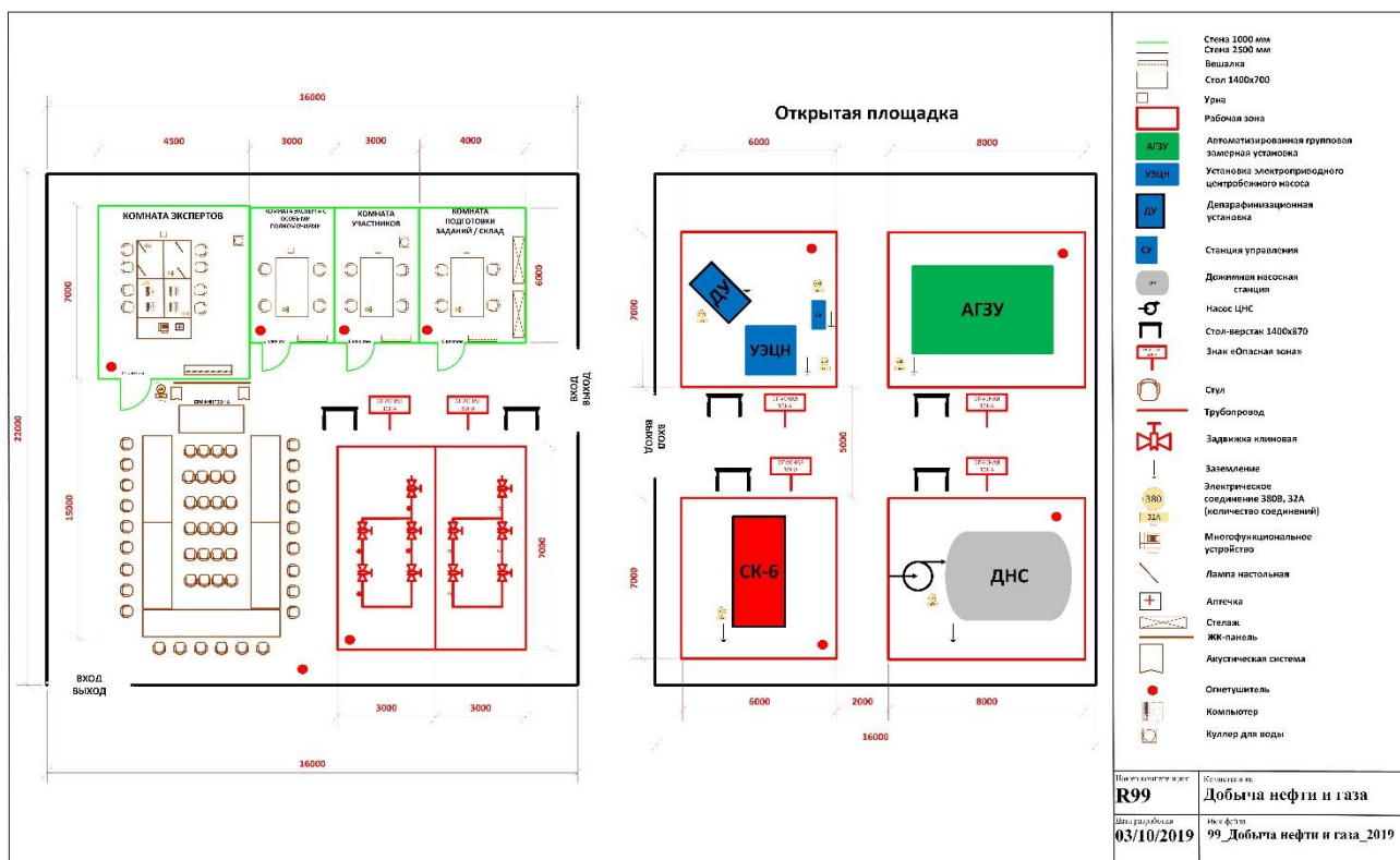
ПЛАН ЗАСТРОЙКИ КОМПЕТЕНЦИИ «ДОБЫЧА НЕФТИ И ГАЗА»
